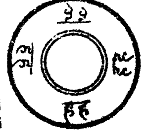
आकाशमंडल
